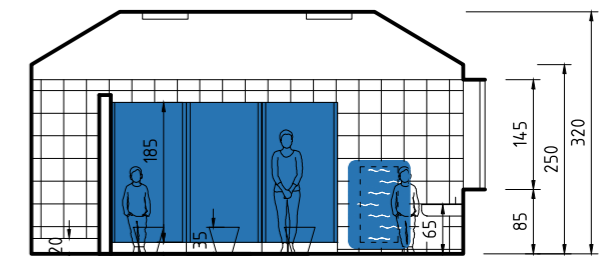
10.B - PRZEKRÓJ
