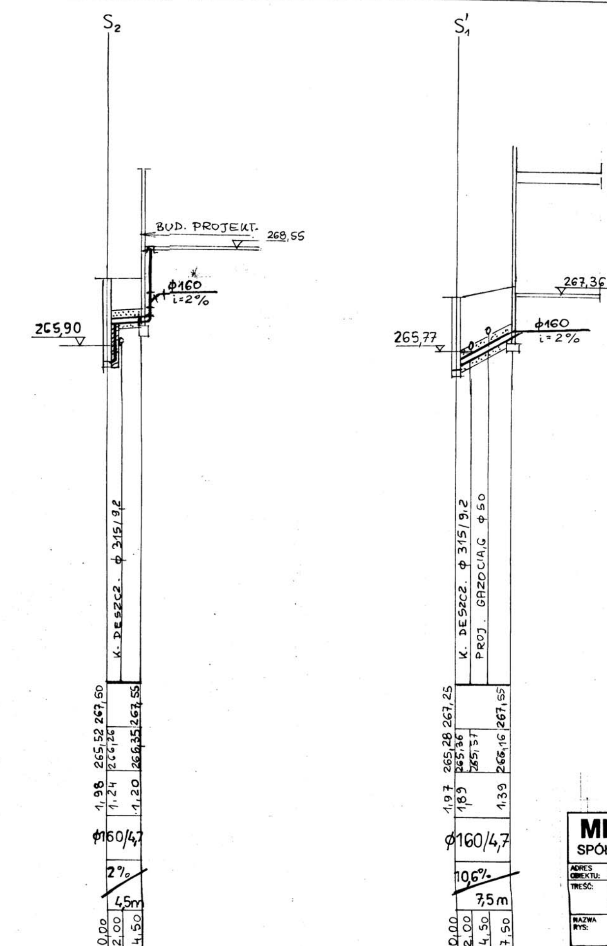
PROFIL PRZYŁĄCZY KAN. SANITARNEJ I PRZEKŁADKI skala 1:500/100
